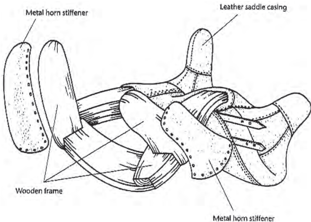
Рис. 45. Реконструкция деревянной основы римского седла (по П. Коннолли)
