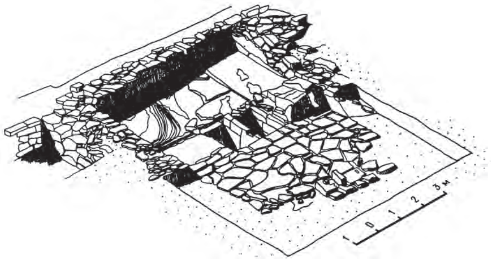
Рис. 6. Производственное помещение илуратской винодельни (аксонометрия)
