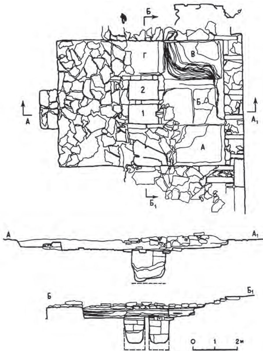
Рис. 5. План и разрезы производственного помещения винодельни
