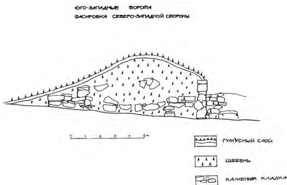
Рис. 19. Фасировка северо-западной стороны единственных сохранившихся ворот Илурата
