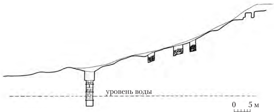
Рис. 17. Разрез склона илуратского плато по линии подземного хода и осадного колодца
