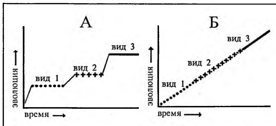
Рис. 2.1. Пунктуалистская (А) и градуалистская (Б) модели макроэволюции.
