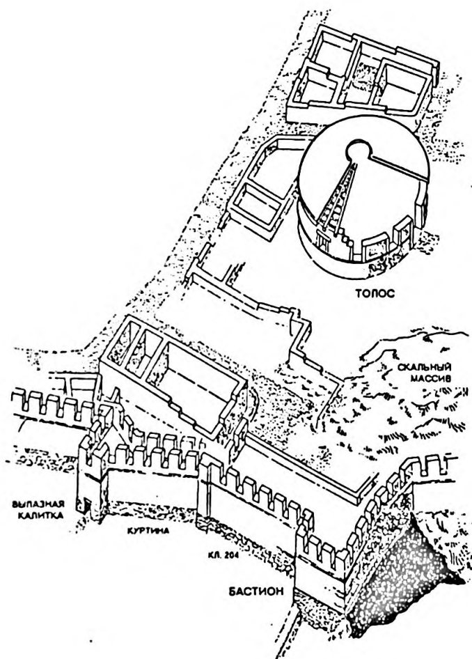
Рис. 15. Укрепления акрополя Пантикапея (по В. П. Толстикову)
