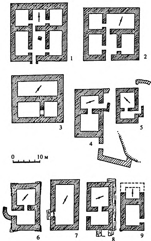
Рис. 40. Планы «домов-башен» Боспора Киммерийского (по Я. М. Паромову)
