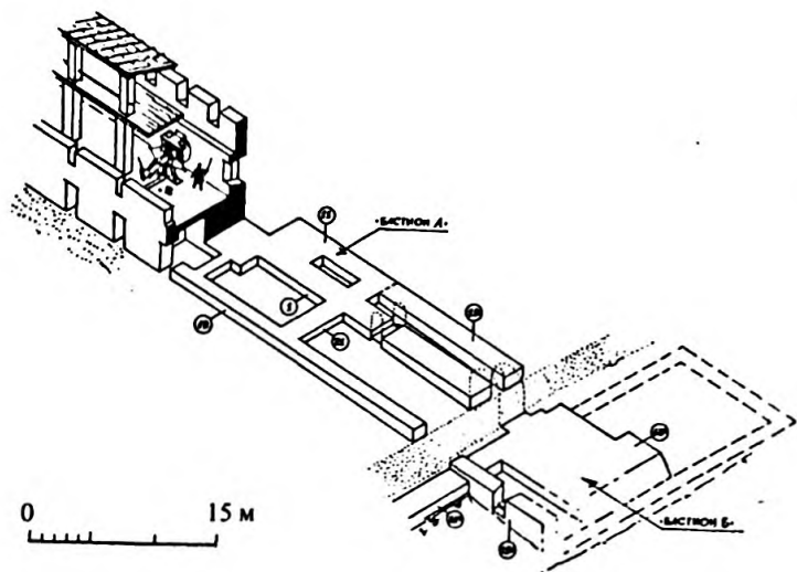
Рис. 42. Акрополь Пантикапея. Куртина, предназначенная для установки катапульт (реконструкция В. П. Толстикова)
