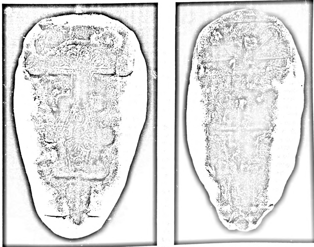
Рис. 11. Экспериментальная глиняная литейная форма. Лицевая и обратная створки
