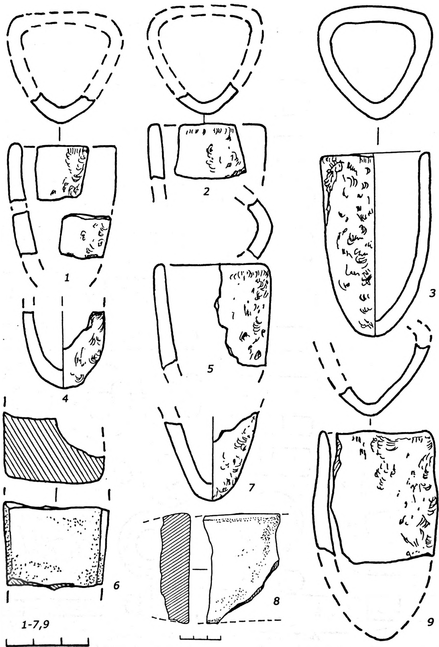
Рис. 8. Тигли и точильные камни поселения Картамышчево II: 1, 5 — яма № 36; 2 — яма № 33; 3, 9 — яма № 38 в жил. 10; 4, 7 — яма № 35; 6, 8 — жил. 7; 1—5, 7, 9 — ошлакованная глина; 6, 8 — песчанник
