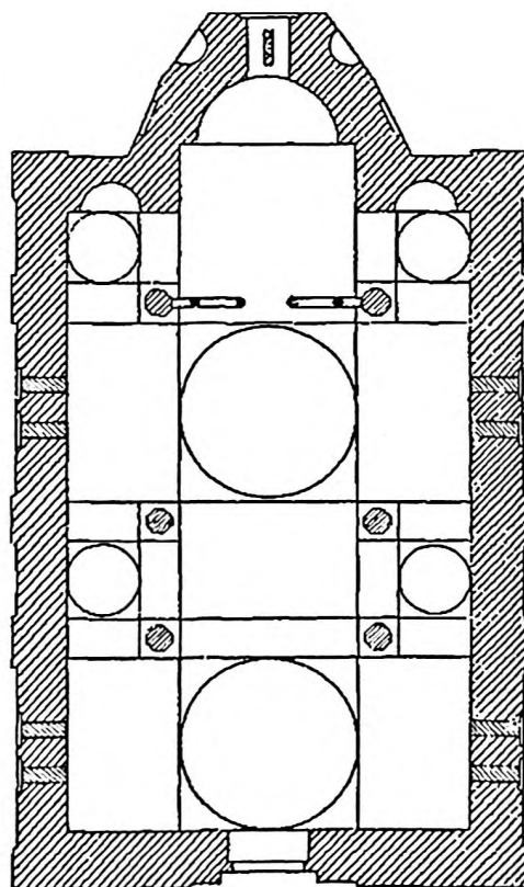
Марков монастырь. План П. П. Покрышкина
