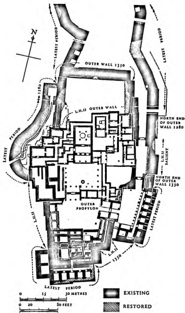
29. Тиринф. План дворца и южной части цитадели (по А. Лоуренсу)
