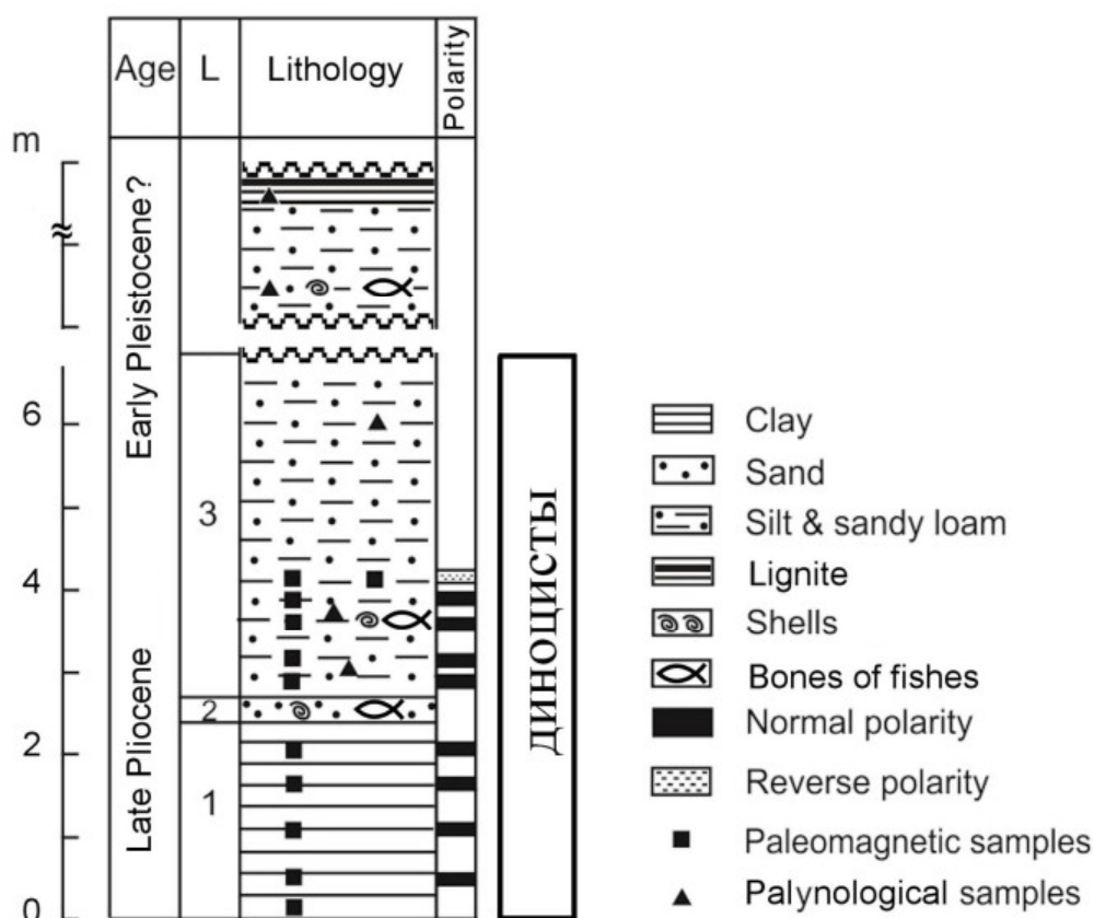
Рис. 4. Разрез отложений верхнего плиоцена — раннего плейстоцена Пекеджик, Турция (по: [Simakova et al., in press])
