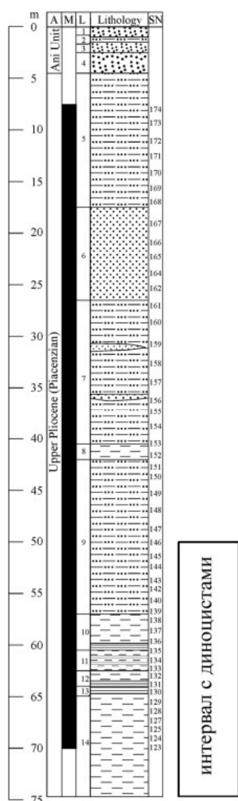
Рис. 3. Разрез отложений верхнего плиоцена — раннего плейстоцена Демиркент, Турция:
