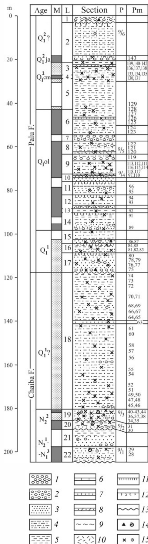
Рис. 6. Разрез отложений плиоцена и нижнего плейстоцена Кованджилар на правом берегу реки Мюрат, Турция:
