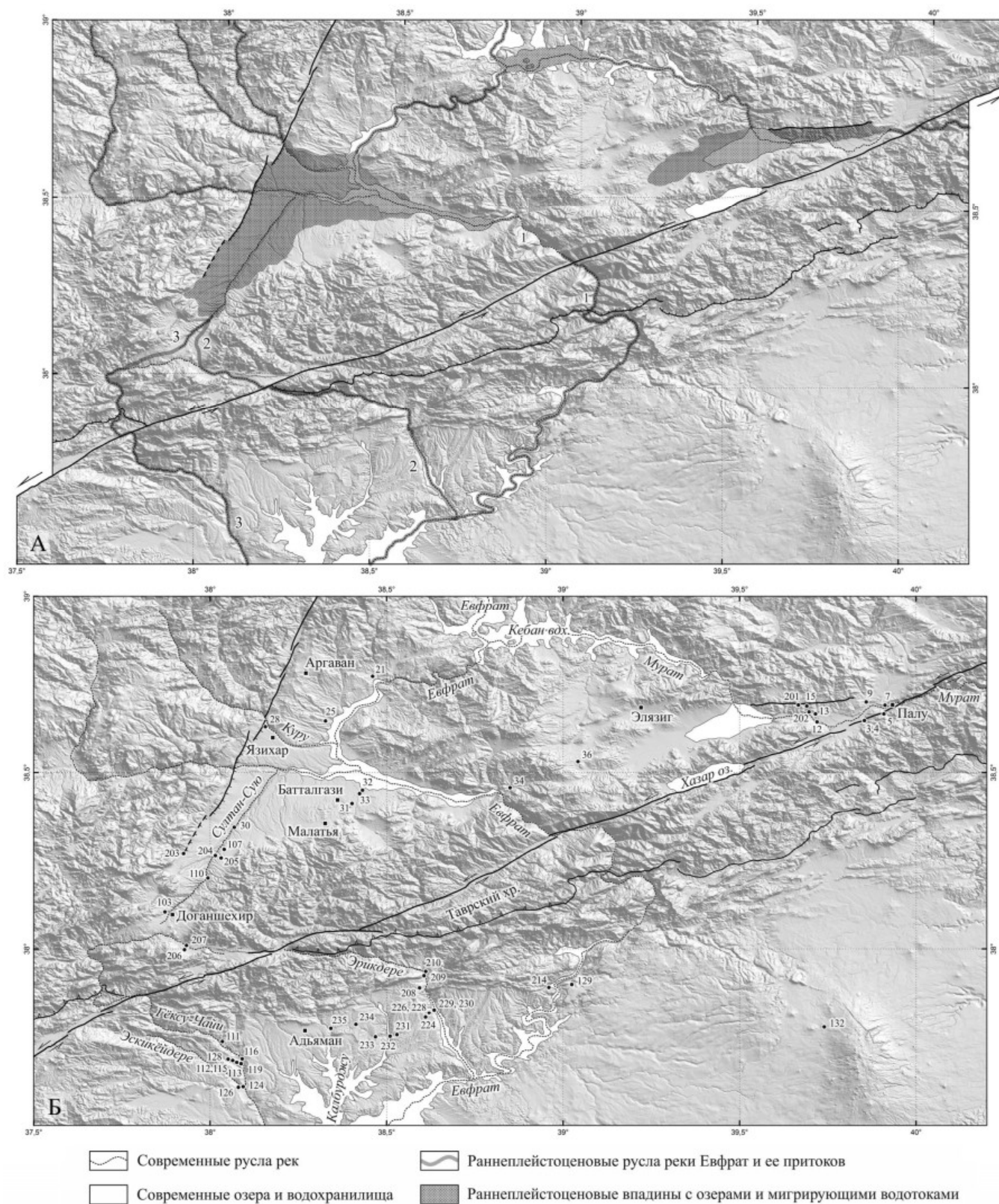
Рис. 9. Изменение местоположения долины р. Евфрата на пересечении с Таврским хребтом (по: [Trifonov et al., 2018]):
