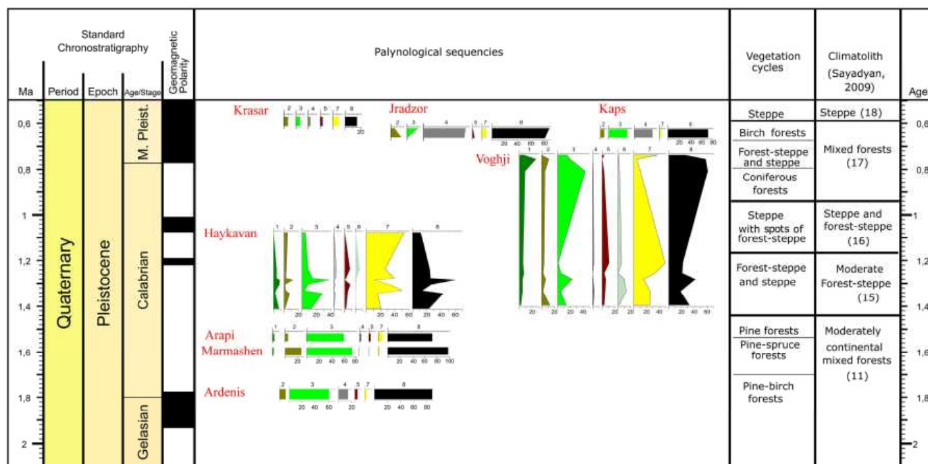
Рис. 7. Палинологическое подразделение отложений конца раннего — начала среднего плейстоцена Ширакской впадины на северо-западе Армении. Стратиграфическое положение и диапазон последовательностей предварительно смоделированы на основе данных Trifonov et al. [2016], Трифонов и др. [2017] и Shalaeva et al. [2019]:
