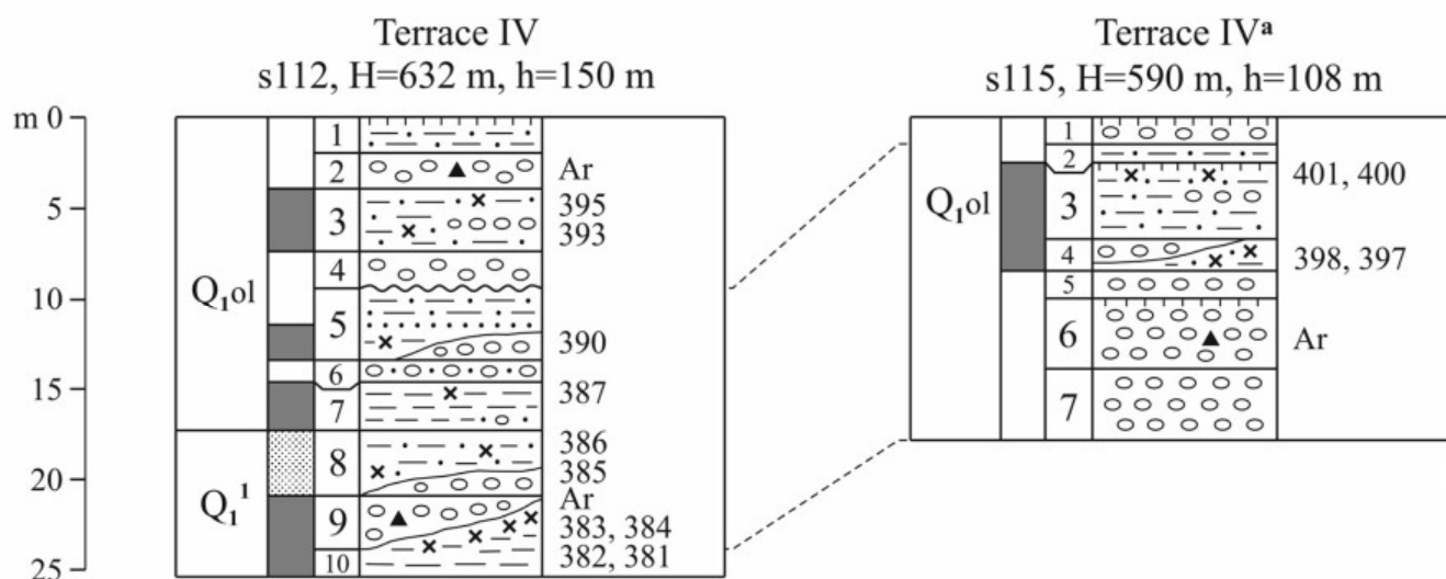
Рис. 5. Разрез отложений плиоцена и плейстоцена Шамбят в долине Гёксу-Чай, Турция. Сопоставление колонок разрезов террас IV и IVa (по: [Trifonov et al., 2018]):
