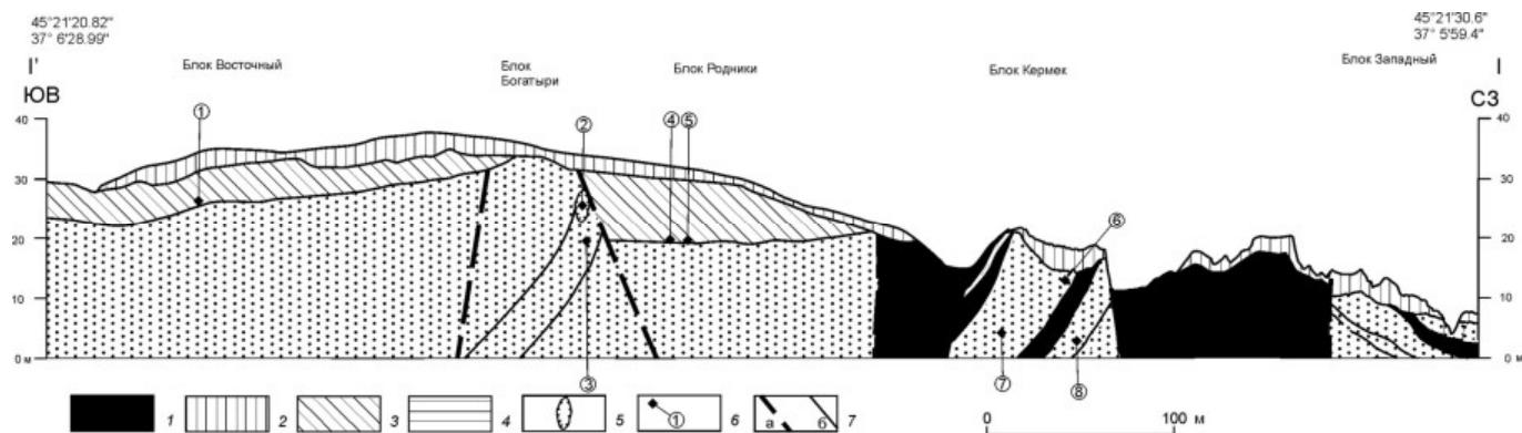
Рис. 2. Геолого-геоморфологический схематический профиль I-I' вдоль береговых обрывов в районе пос. За Родину на северо-востоке Таманского п-ва (по: [Тесаков и др., 2019]). Палеонтологические и археологические местонахождения:
