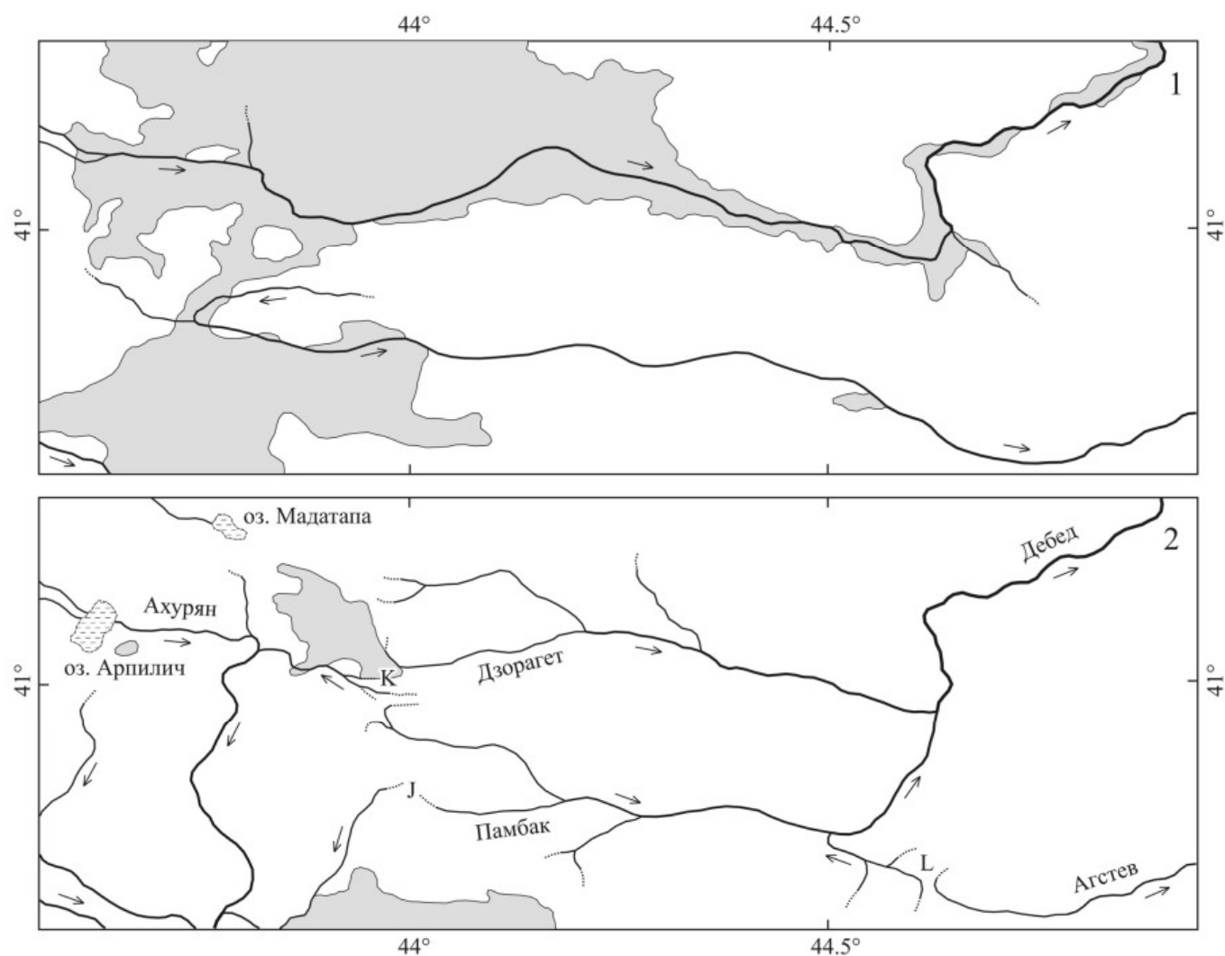
Рис. 8. Изменения дренажной сети на севере Армении в четвертичное время:
